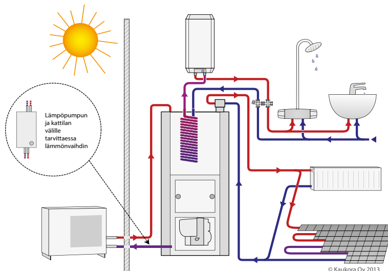
Jäspi VLK kytkettynä öljykattilaan ja ilma-vesilämpöpumppuun
