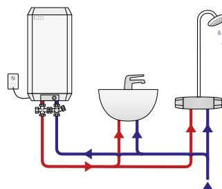
Jäspi VLK lämmitää talouden käyttöveden
